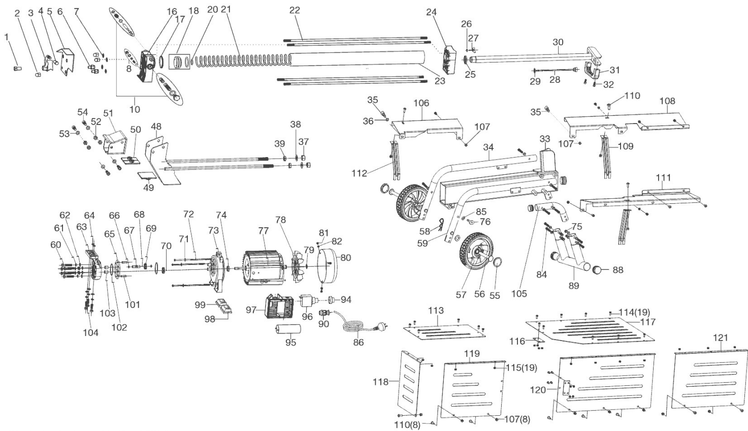
O.-Abb. Schraubenbeutel Art.-Nr. 419066
